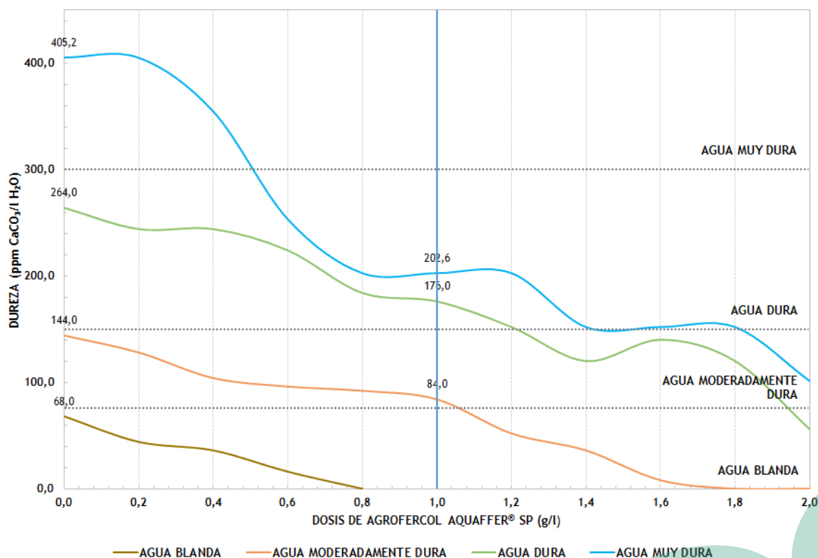
CURVA DE DUREZA AGROFERCOL AQUAFER® SP
